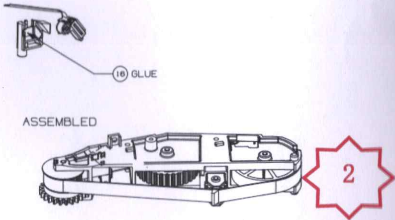
图二，PA04160 组件，带铁氧体线圈组件
